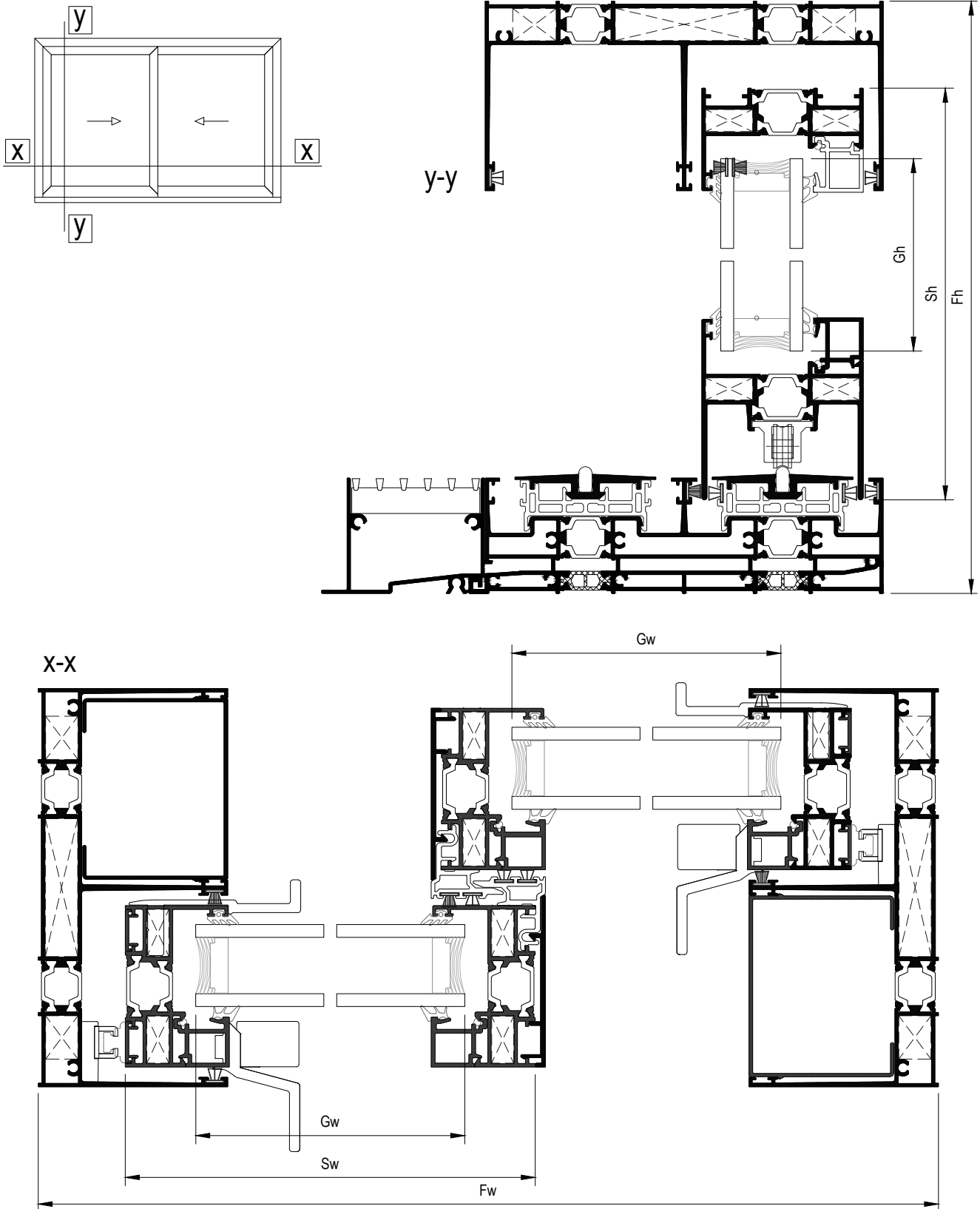
Ag Two-sash sliding window with gutter Δίφυλλο επάλληλο συρόμενο με υδατολεκάνη
