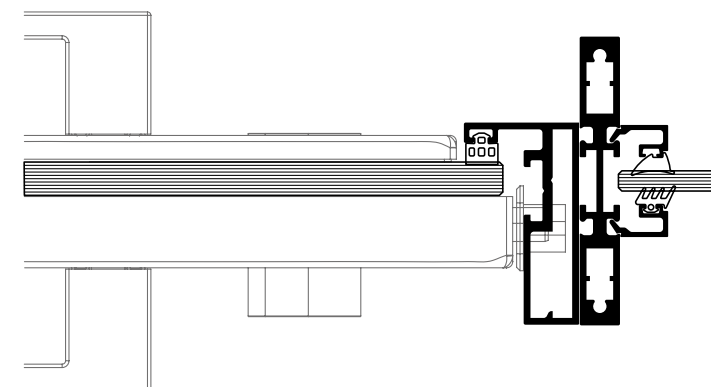
ΛΕΠΤΟΜΕΡΕΙΑ ΚΛΕΙΔΩΜΑΤΟΣ
