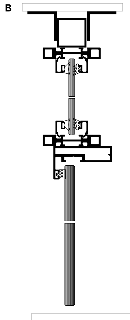
Κάθετη τομή πόρτας με φεγγίτη
