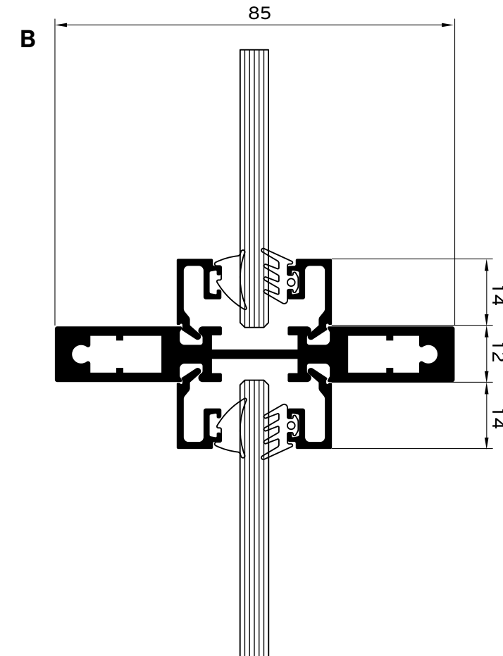
Κατακόρυφη τραβέρσα
